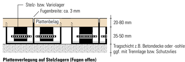
Plattenverlegung auf Stelzlager (Fugen offen)
