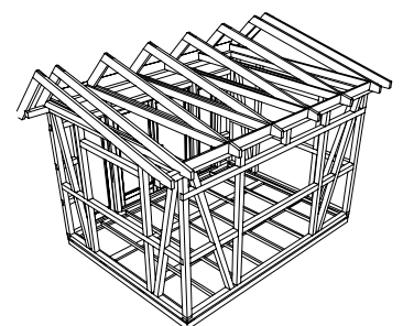
Grundgerüst 4 x 3 m
